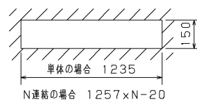
N連結の場合 1257×N-20 埋込み穴寸法
