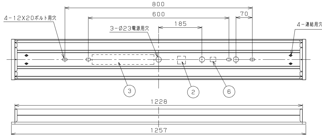
N連結の場合 1257xN-20 埋込み穴寸法
