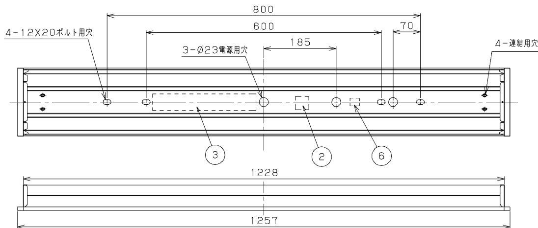
N連結の場合 1257 \times N - 20 埋込み穴寸法
