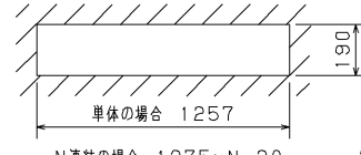
N連結の場合 1275×N-20 埋込み寸法
