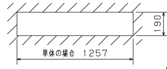
N連結の場合 1275×N-20 埋込み寸法
