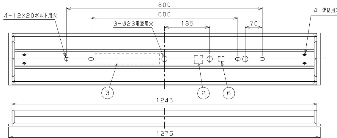
N連結の場合 1275×N-20 埋込み寸法
