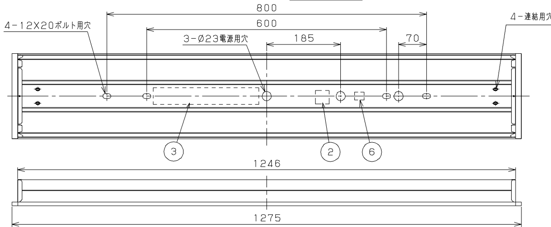
単体の場合 1257 N連結の場合 1275×N-20 埋込み寸法
