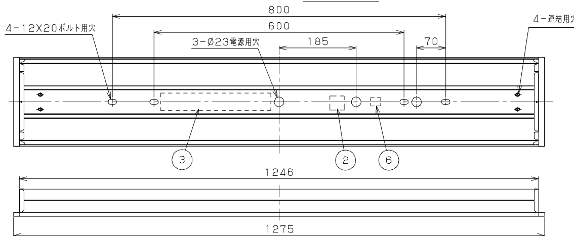
N連結の場合 1275 \times N - 20 埋込み穴寸法
