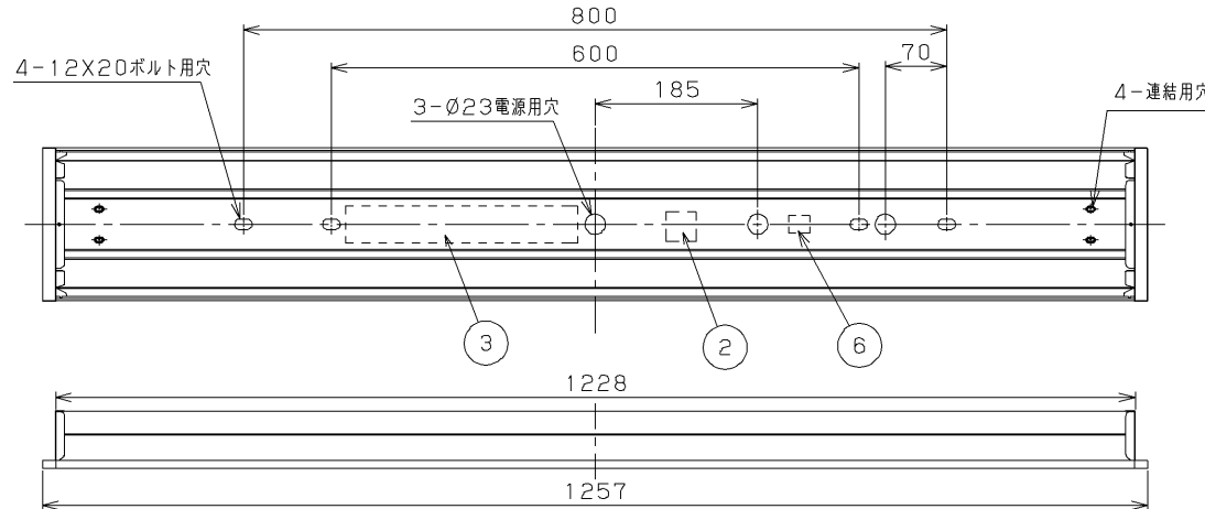
N連結の場合 1257×N-20 埋込み穴寸法
