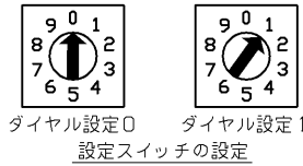
設定スイッチの設定
