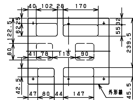
配線寸法
