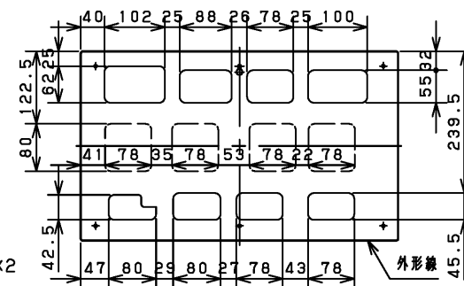
配線穴寸法
