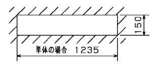
埋込み寸法
