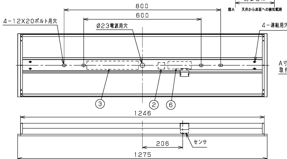
図B 床面検知範囲
