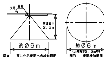
図A 天井から床面への検知範囲
