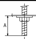
取付ボルトを使用した場合の器具内寸法
