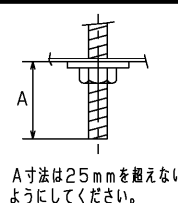
取付ボルトを使用した場合の器具内寸法
