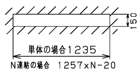
埋込み寸法
