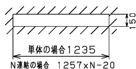
埋込み穴寸法
