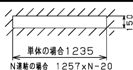
埋込み寸法
