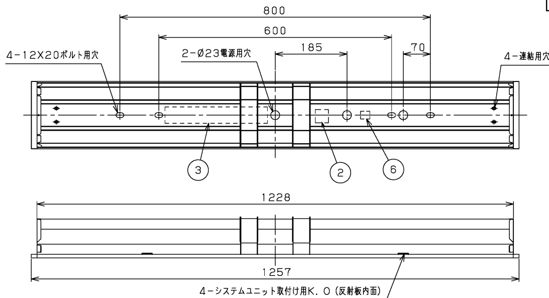
取付ボルトを使用した場合の器具内寸法
