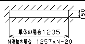
埋込み寸法
