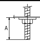
取付ボルトを使用した場合の器具内寸法
