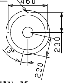
取付けピッチ寸法図 4-φ4.5木ねじ用K.0
