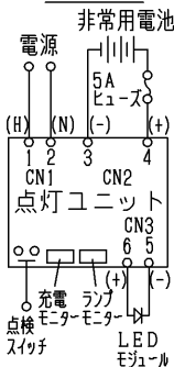
結線図
