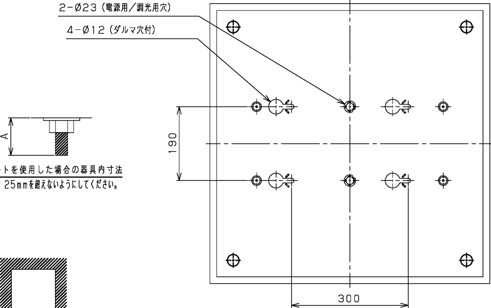
埋込み取付けの場合の埋込み寸寸法
