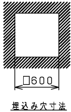
埋込み寸法
