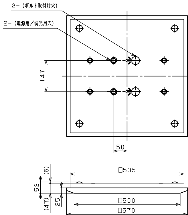
取付けボルトを使用した場合の器具内寸法
