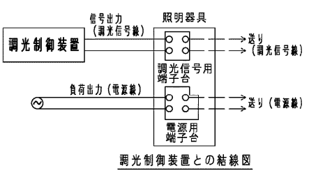
調光制御装置との結線図
