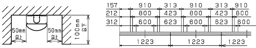
直付け連結使用例
