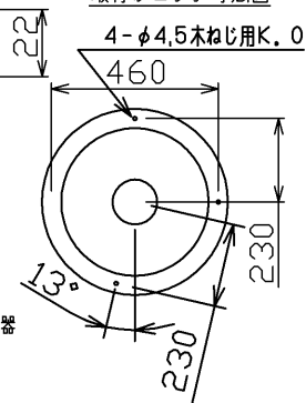
取付けピッチ寸法図
