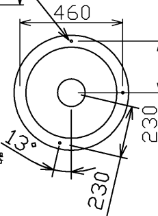
取付けピッチ寸法図 4-φ4.5木ねじ用K.0
