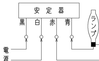
結線図
