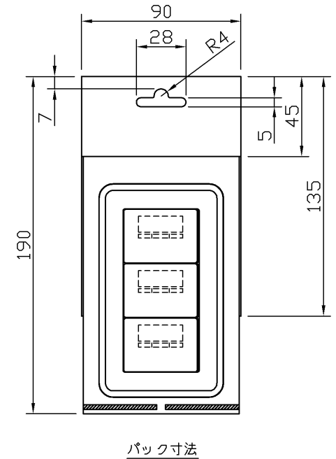
パック寸法
