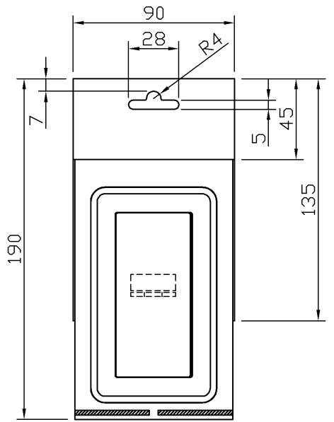
バック寸法
