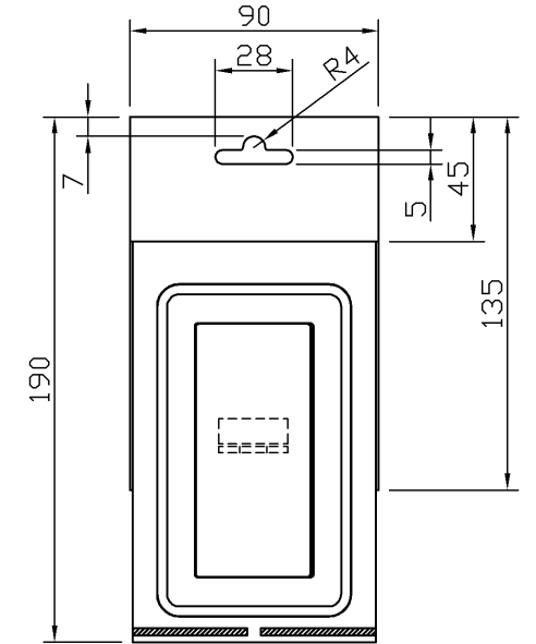
パック寸法
