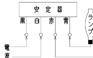
結線図
