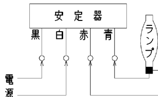
結線図
