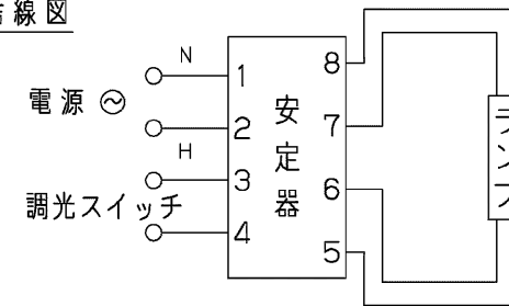
結線図
