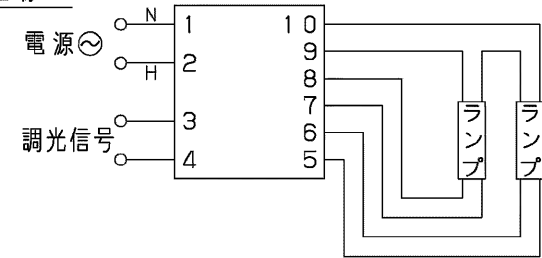
結線図
