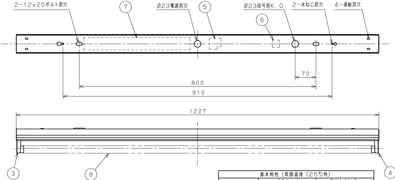
取付けボルトの器具内寸法
