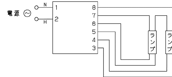
結線図
