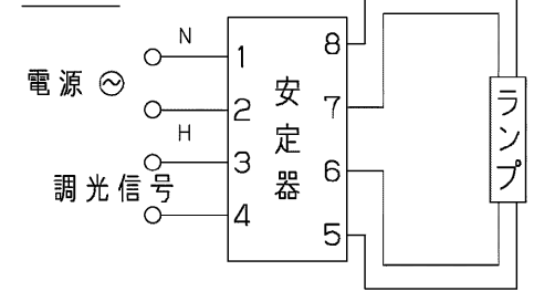
結線図
