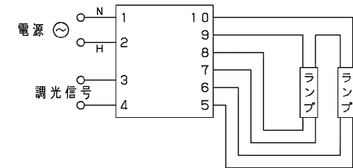
結線図
