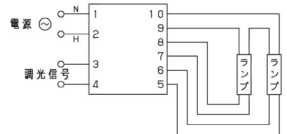
結線図
