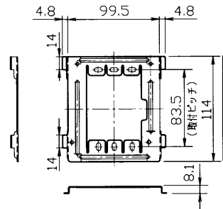
取付金具(t1.2)
