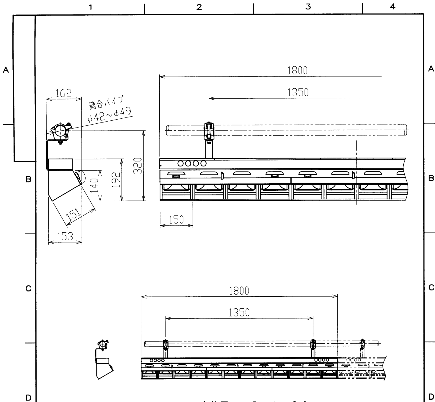
全体図 S = 1 / 20
