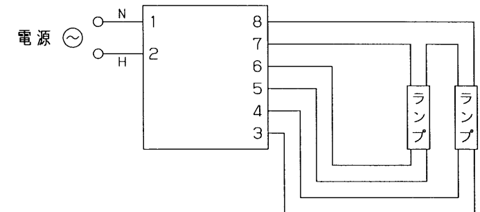
結線図
