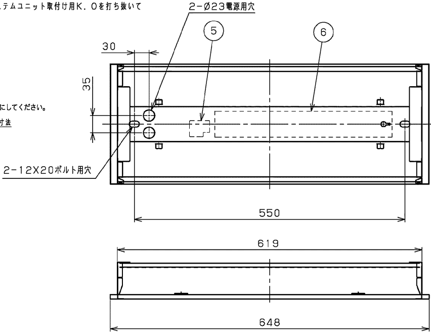
FHF 32器具N連結+FHF 16器具の場合 1257×N+628 埋込み穴寸法
