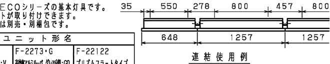
連結使用例
