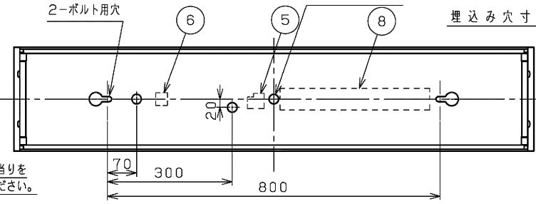
N連結の場合 1251×N-16
