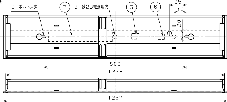
N連結の場合 1257×N-20 埋込穴寸法
