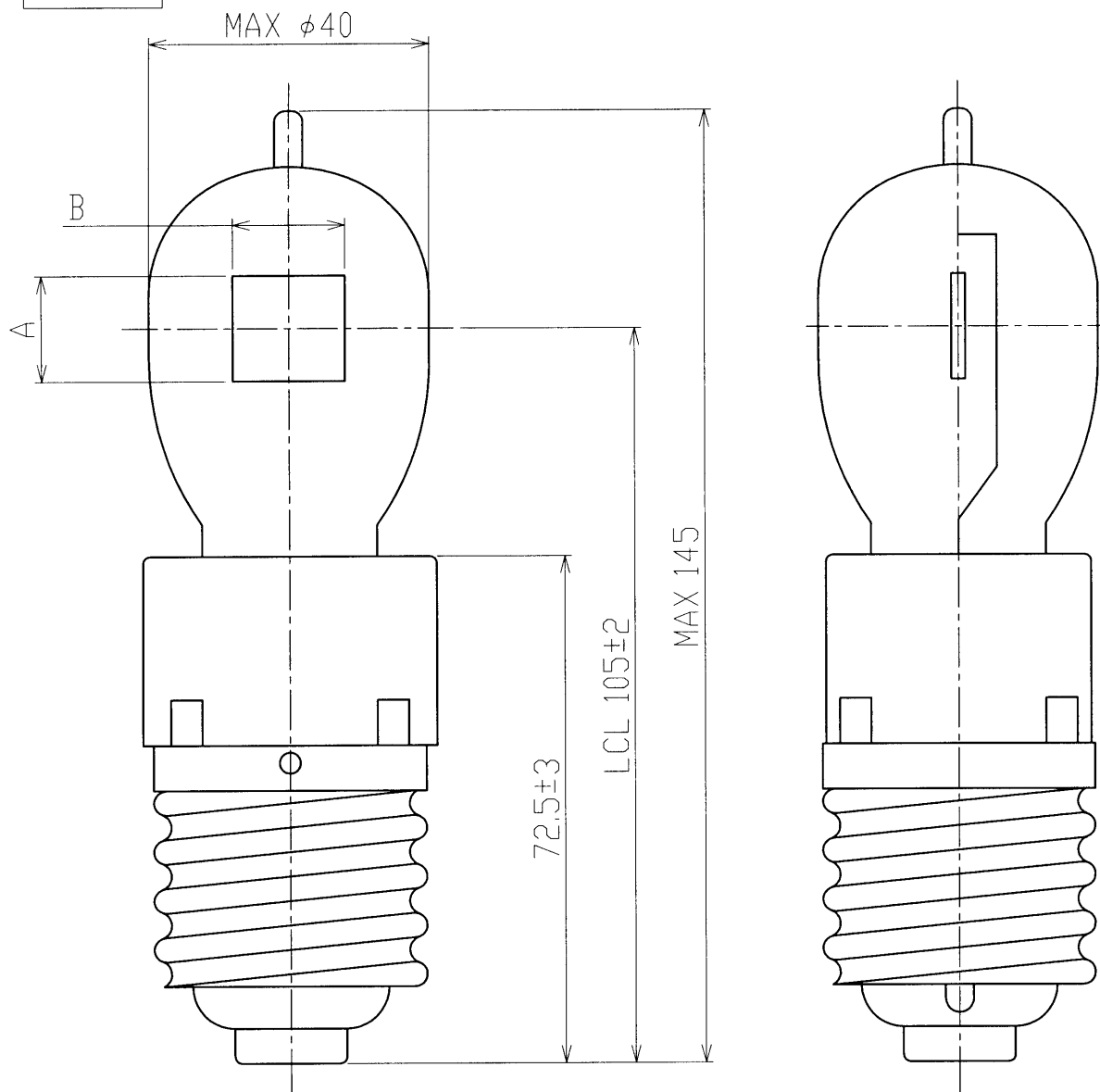
外形図
